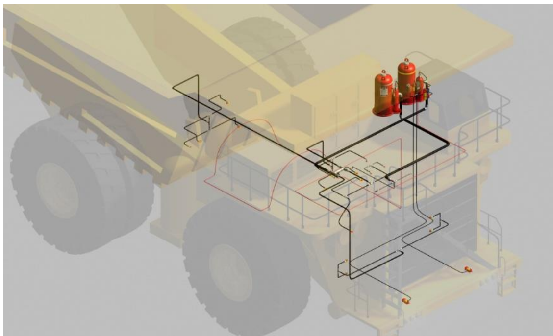
Рис. 1. Расположение двухкомпонентной системы пожаротушения ANSUL
